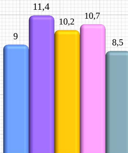
модуль "Алгебра"
