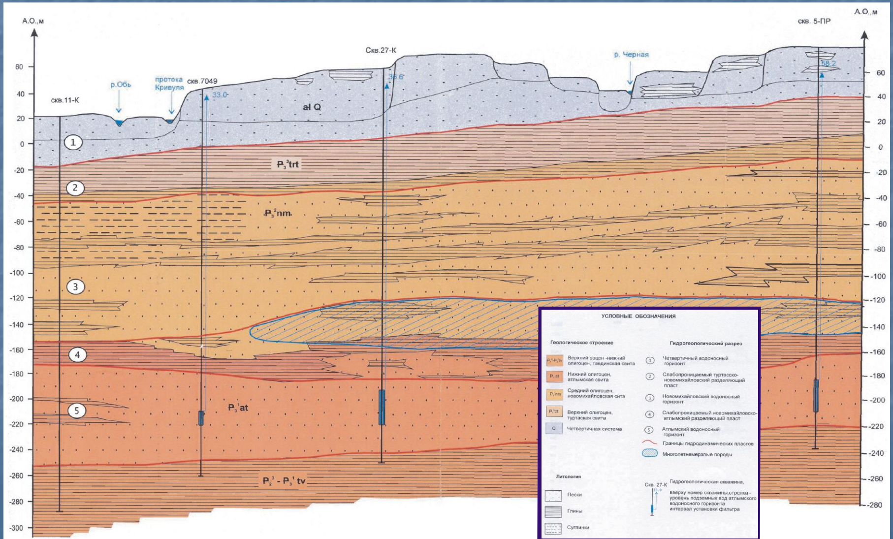
Рис. 14. Схема расположения водоносных горизонтов подземных вод на территории г. Сургута
