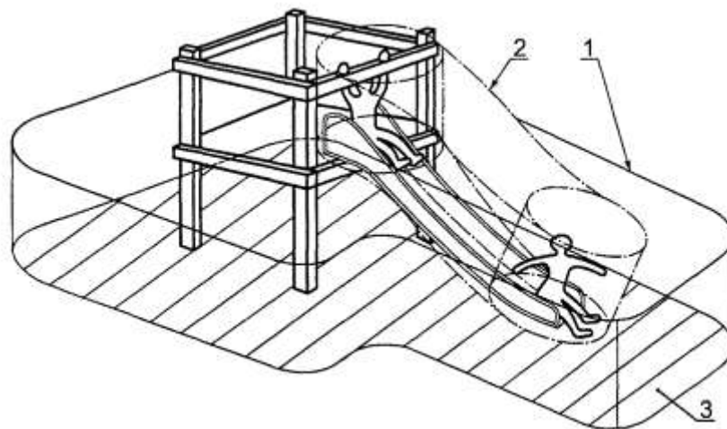
1 - игровая зона; 2 - зона безопасности; 3 - зона приземления
