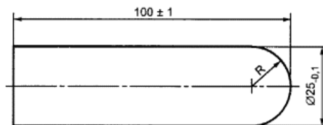
Рисунок Г.12 - Стержень-палец А (малый)
