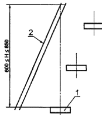
Рисунок 7 - Перила для лестниц
