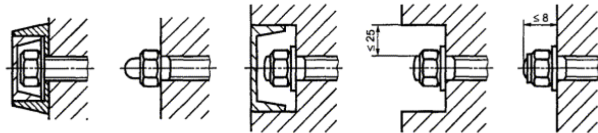
Рисунок 4 - Защита болтовых соединений
