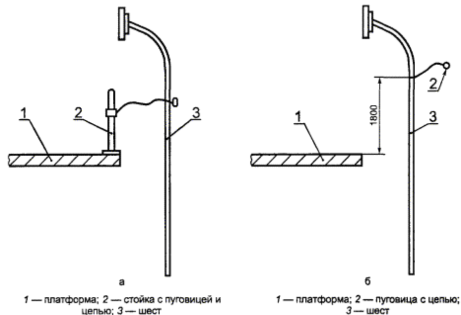
Рисунок Г.11 - Испытания шеста
