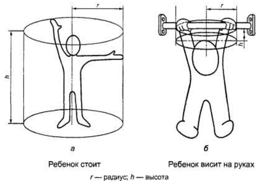
Рисунок 11 - Размеры цилиндра для определения зоны безопасности
