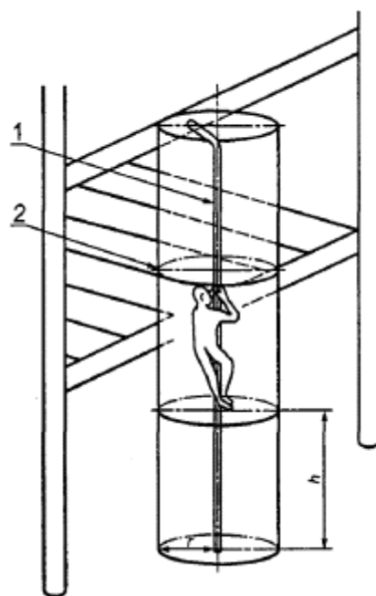
Рисунок 10 - Определение зоны безопасности шеста
