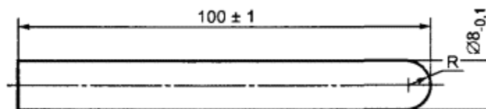
Рисунок Г.12 - Стержень-палец А (малый)
