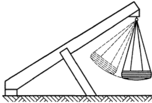
Рисунок А.3 - Качающаяся платформа
