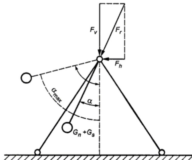
Рисунок А.2 - Силы, действующие на качели
