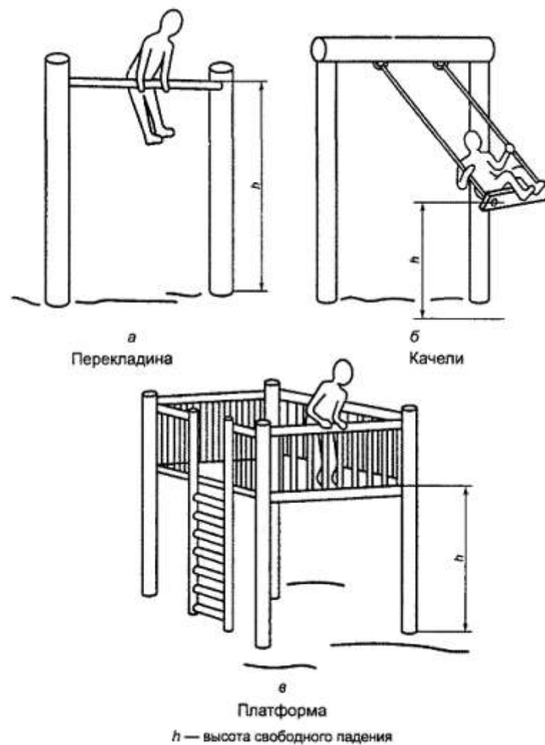
Рисунок 13 - Высота свободного падения h для различного оборудования
