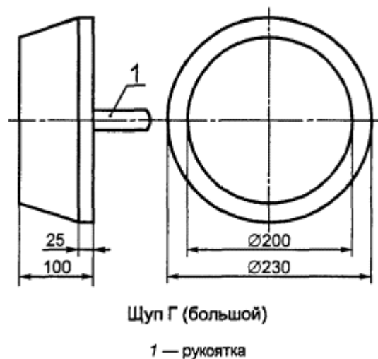
Рисунок Г.3 - Щуп Г (большой) для определения застревания головы или шеи в отверстиях
