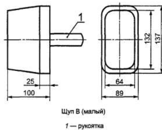
Рисунок Г.2 - Щуп В (малый) для определения застревания головы или шеи в отверстиях
