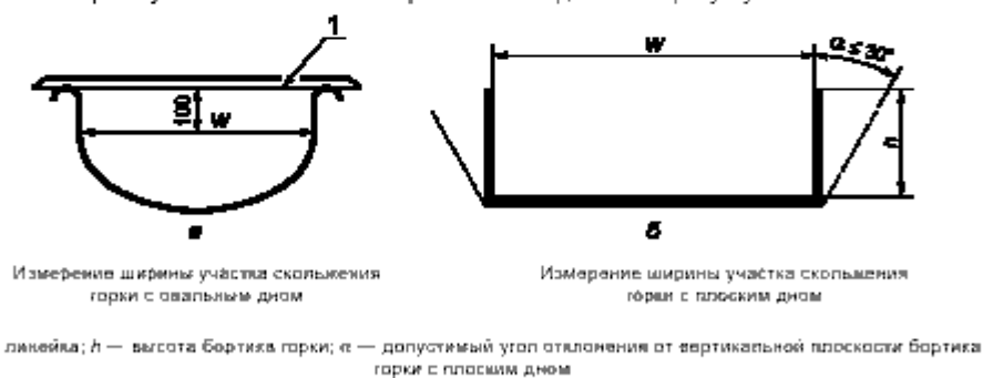
Рисунок А.1 — Измерение ширины участка скольжения горки
