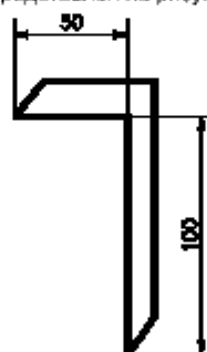
Рисунок А.3 — Шаблон для измерения профиля горки
