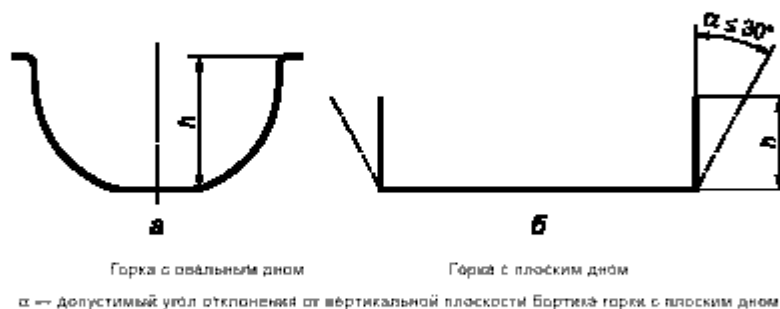
Рисунок 9 — Профили горки
