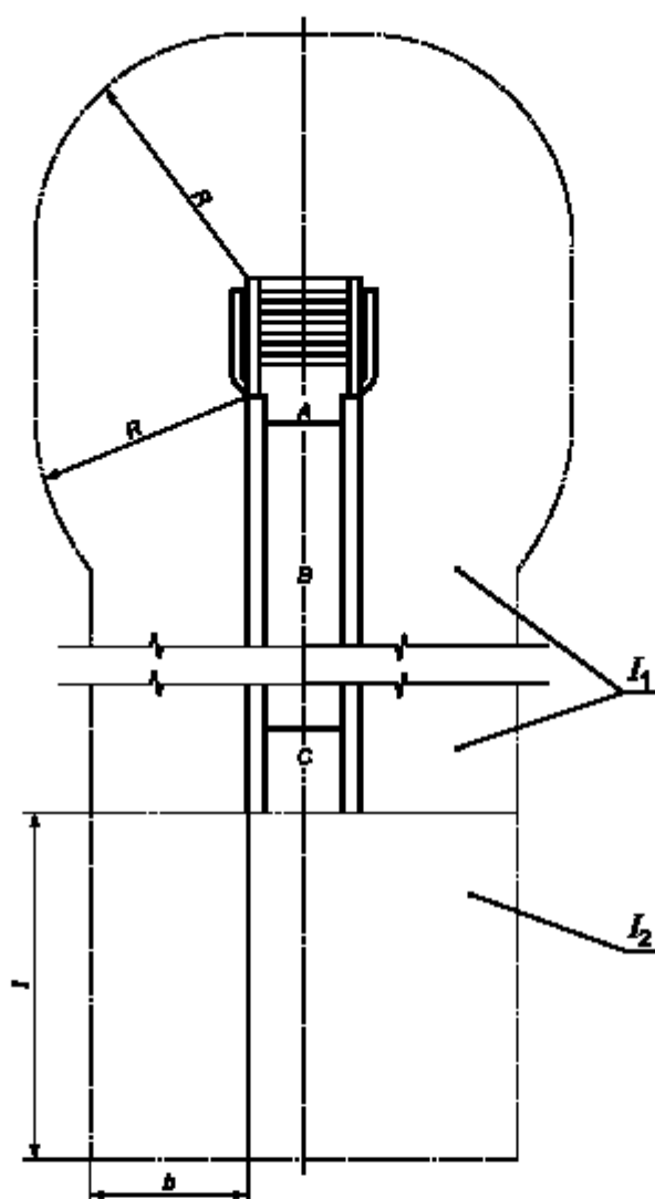
А — стартовый участок; В — участок скопления; С — конечный участок; b — ширина зоны приземления; R — радиус зоны приземления; L_1 — зона приземления по бокам горки; L_2 — зона приземления в конечном участке горки; L — длина зоны приземления в конечном участке горки
